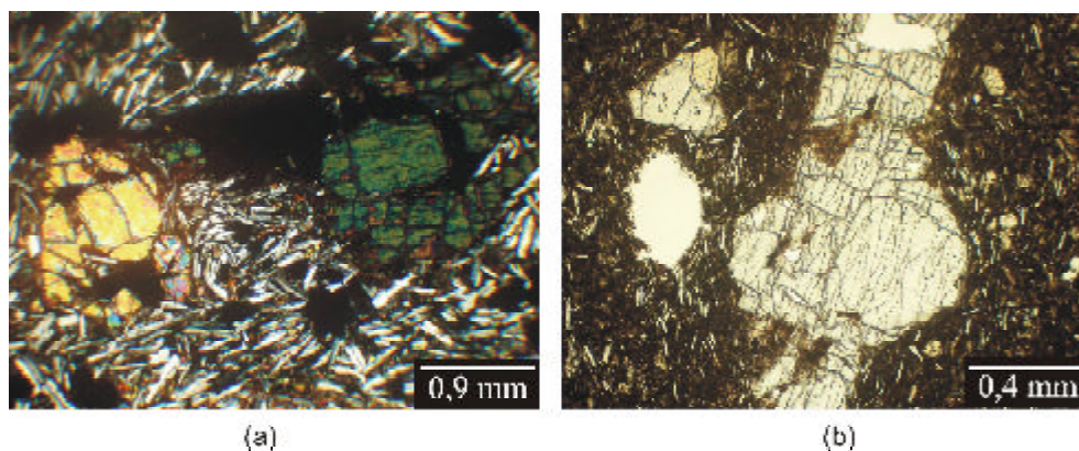
Fig. 14: textura inequigranular. (a) bimodal (fenocristales de olivino en matriz de plagioclase, piroxenos y minerales opacos, basalto, Nx), (b) trimodal (fenocristal de piroxeno y matriz con microclitos de plagioclase y material afanítico, basalto, N//).
