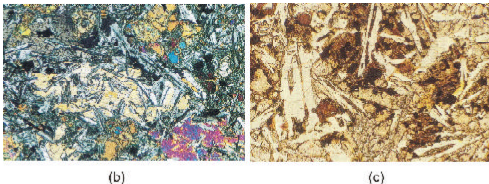
Fig. 41: (b) textura subofítica. Cristales de plagioclasa incluidos total y parcialmente en cristales de augita (dolerita olivínica Nx y N//, x 27); (c) textura hialofítica. Cristales de plagioclasa rodeados por vidrio desvitrificado de color pardo oscuro (basalto oceánico N//, x65).
