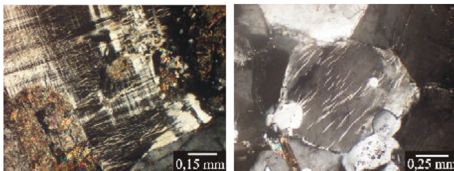
Fig. 29: cristales de microclino pertítico (granito, Nx)
