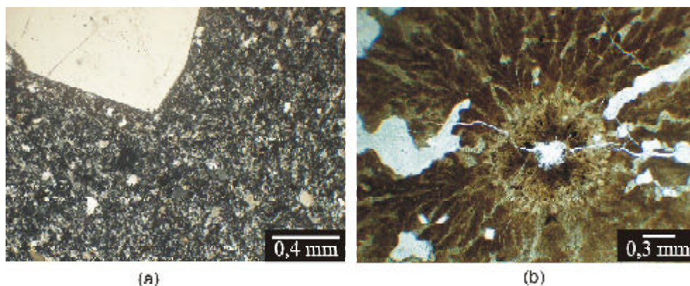
Fig. 37: (a) matriz con textura felsítica (dacita, Nx). (b) textura esferulítica: esferulita de feldespato alcalino formada por desvitrificación de vidrio volcánico (N//).
