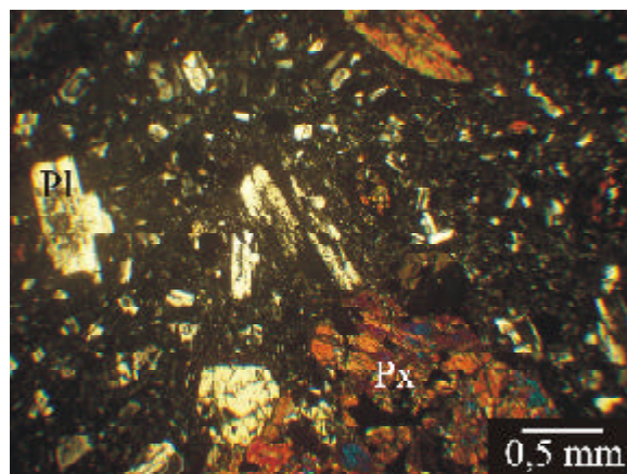
Fig. 11: (a) distribución trimodal del tamaño de grano (basalto, Nx)
