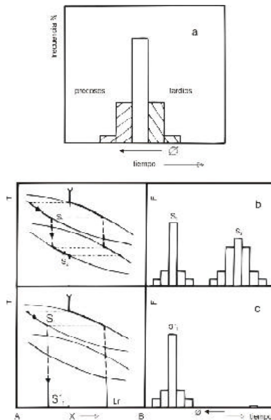
Fig. 10: (a) variación del tamaño ( \phi ) de los cristales con el tiempo en sistemas donde son homogéneas las velocidades de nucleación y crecimiento cristalino, existen entonces tres poblaciones de cristales de tamaño variable. (b) cristalización de una solución sólida a partir de un líquido L en un sistema que experimenta un cambio brusco de T y/o de P; existen entonces dos poblaciones de cristales en los cuales los minerales tienen tamaños variables. (c) igual situación que la anterior con fuerte descenso de T y/o P (caso de lavas)
