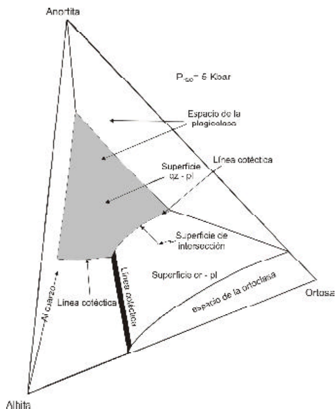
Fig. 7: sistema granítico cuaternario (modificado de Hibbard, 1995).
