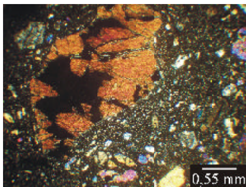
Fig. 6: ejemplo de cristalización en tres etapas: dos tamaños de fenocristales de piroxenos y una matriz afanítica (basalto, Nx)
