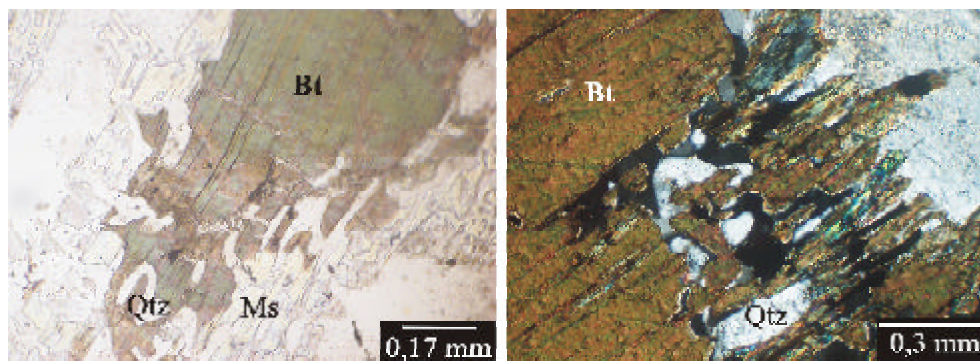
Fig. 26: Textura simplectítica (granitos, N// y Nx).
