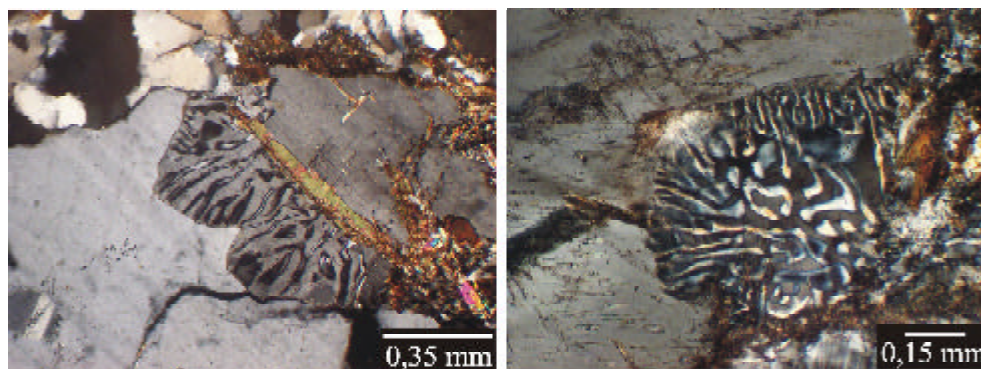
Fig. 28: Textura mirmequítica en granitos (Nx).
