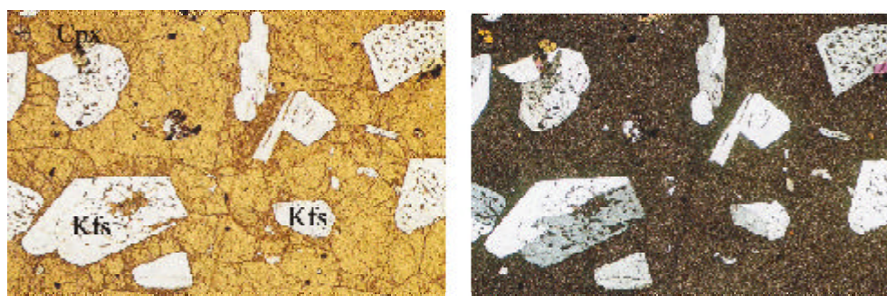
Fig. 9 (b): textura merocristalina. Fenocristales de Feldespato Potásico (Kfs) y pequeños cristales de clinopiroxenos (Cpx) en una matriz microcristalina a vítrea con textura perlítica (riolita x7, N// y Nx)
