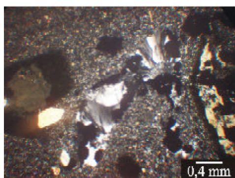
Fig. 46 (b) las vesículas originales de este basalto están rellenas por zeolitas (Nx); y (c) las vesículas están rellenas en parte por piroxenos (Nx y N//).
