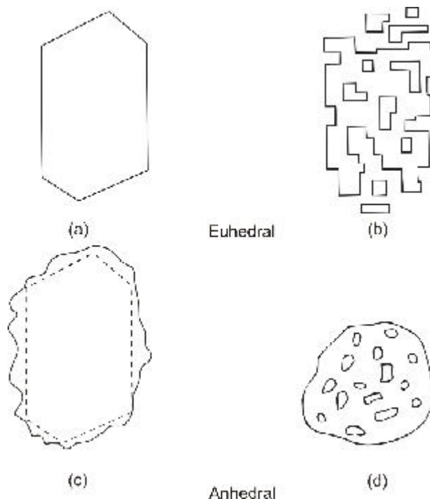
Fig. 19: esquema de cristales que muestran la limitación de la clasificación de “forma de los cristales” tradicional. Los cristales (a) y (b) son muy diferentes (a) está completo y (b) es celular, pero ambos están totalmente limitados por caras cristalinicas, lo que satisface el criterio de “euhedral”. Los cristales (c) y (d) son muy diferentes (c es casi euhedral, d está lejos de serlo), pero ambos carecen de caras cristalinicas, lo que satisface el criterio de “anhedral”.
