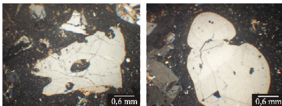
Fig. 16: cristales de cuarzo con bordes corroídos (dacita, Nx).
