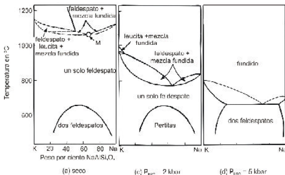
Fig. 32: diagrama de fases para el sistema albita - ortosa (Modificada de Bowen y Tuttle, 1950).
