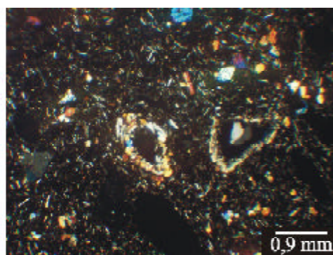
Fig. 46 (b) las vesículas originales de este basalto están rellenas por zeolitas (Nx); y (c) las vesículas están rellenas en parte por piroxenos (Nx y N//).
