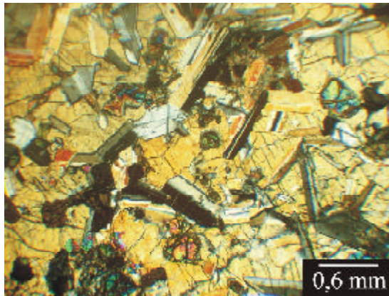
Fig. 41: (a) textura ofítica: cristal de augita encierra a numerosos cristales de Plagioclase dispuestos al azar (gabro, Nx)
