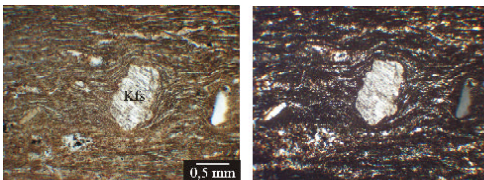
Fig. 43: Textura de flujo (riolita, N // y Nx).
