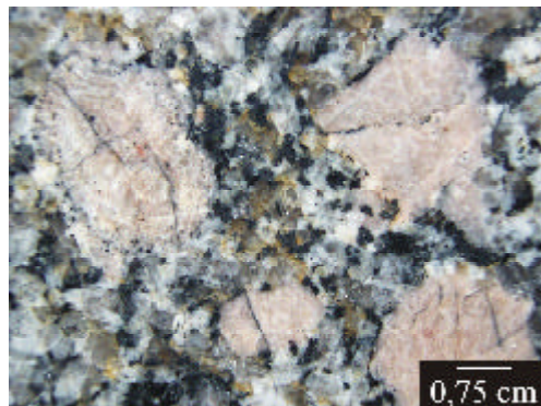
Fig. 8: muestra de mano pulida de un granito porfirico con megacrystales de Feldespato Potásico.
