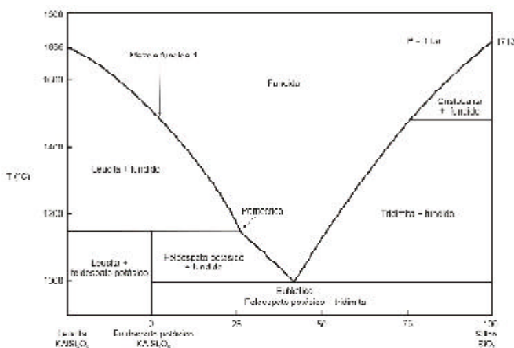
Fig. 1: Sistema de fusión incongruente leucita-sílice (Modificado de Schairer y Bowen, 1947)
