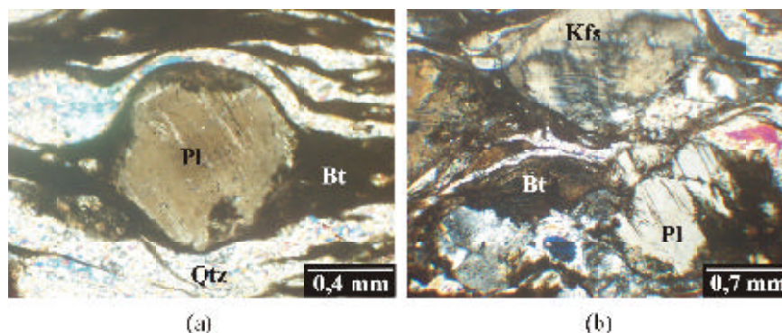
Fig. 18: texturas dúctiles. (a) porfiroclasto con estructura asimétrica (Nx), (b) mica fish y microclino con maclado anómalo (Nx).
