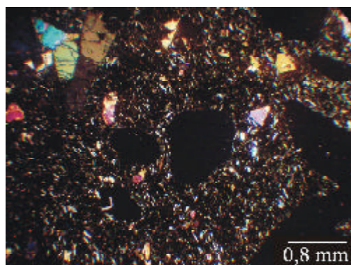
Fig. 46: (a) estructura vesicular. Cavidades subesféricas distribuidas aleatoriamente en un basalto (Nx y N//)
