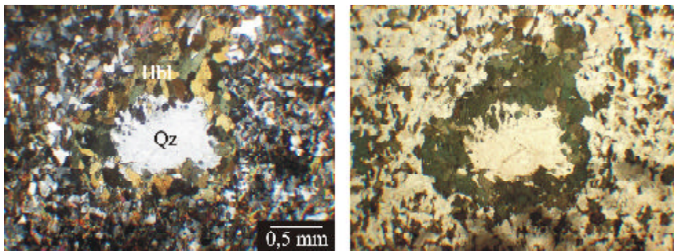
Fig. 36 (b) textura ocelar: xenocristal de cuarzo rodeado de numerosos cristales de hornblenda (diorita, Nx y N//).
