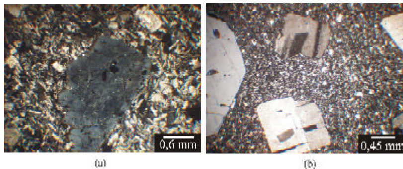
Fig. 5: ejemplos de cristalización en dos etapas: Los fenocristales cristalizaron previamente a la matriz. (a) traquita (Nx), (b) dacita (Nx).
