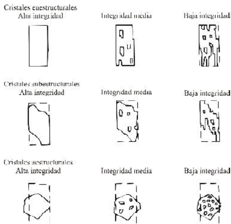
Fig. 20: clasificación morfológica de los cristales (modificado de Hibbard, 1995).
