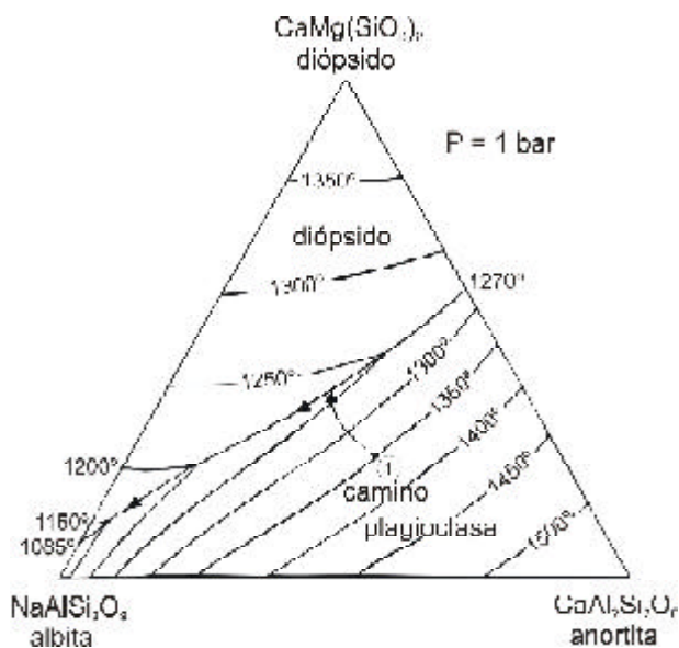
Fig. 42: diagrama del sistema albita - anortita - diópsido (traducido de Hibbard, 1995).
