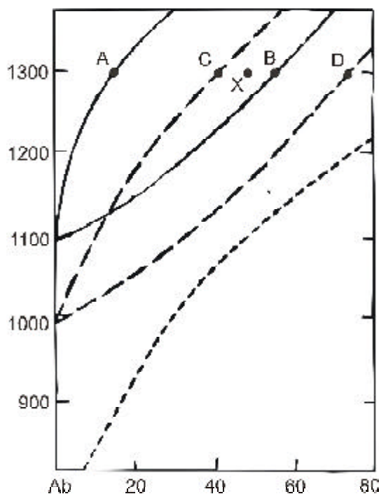
Fig. 25: diagrama de fases para el sistema albíta - anortita. Sistema anhidro (líneas llenas) comparado con el sistema a presión de agua a 5000 bars (línea de trazos cortos, inferior derecha). Las líneas de trazos representan hipotéticamente una presión de agua intermedia. (Modificado de Turner y Verhoogen, 1978)
