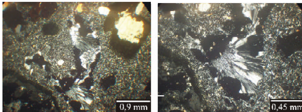
Fig. 37: (c) esferulitas de zeolitas relleno de vesículas de un basalto (Nx).
