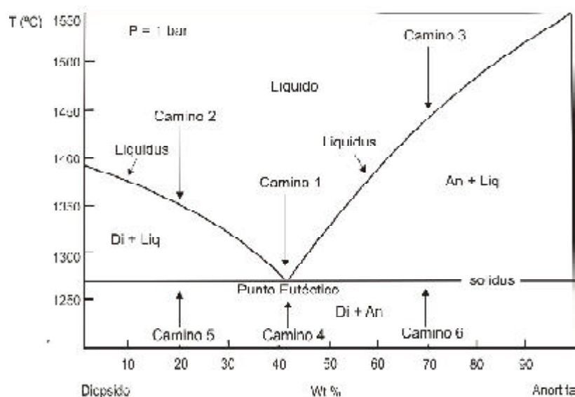
Fig. 27: sistema diópsido - anortita (fusión con punto eutéctico, modificado de Hibbard, 1995).
