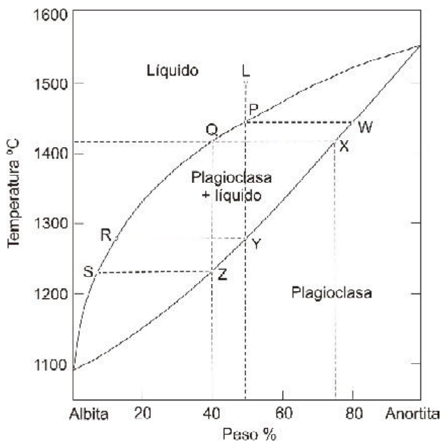
Fig. 23: diagrama de fases para el sistema albita - anortita (sistema anhidro a presión atmosférica) Modificado de Bowen, 1913.
