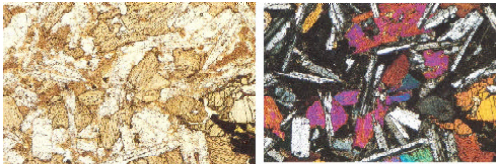
Fig. 40: textura intersertal. Cristales de plagioclase rodeados de analcima (incolores con N// e isótropa con Nx), otras plagioclases están parcialmente incluidas en piroxeno (dolerita x23. N// y X).
